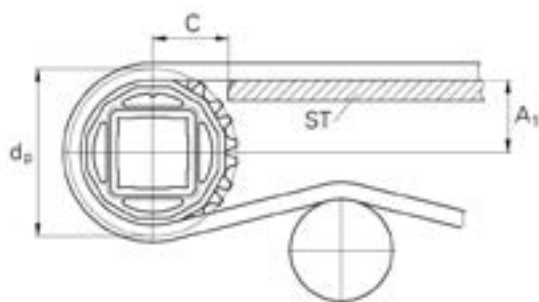
Drive sprocket
